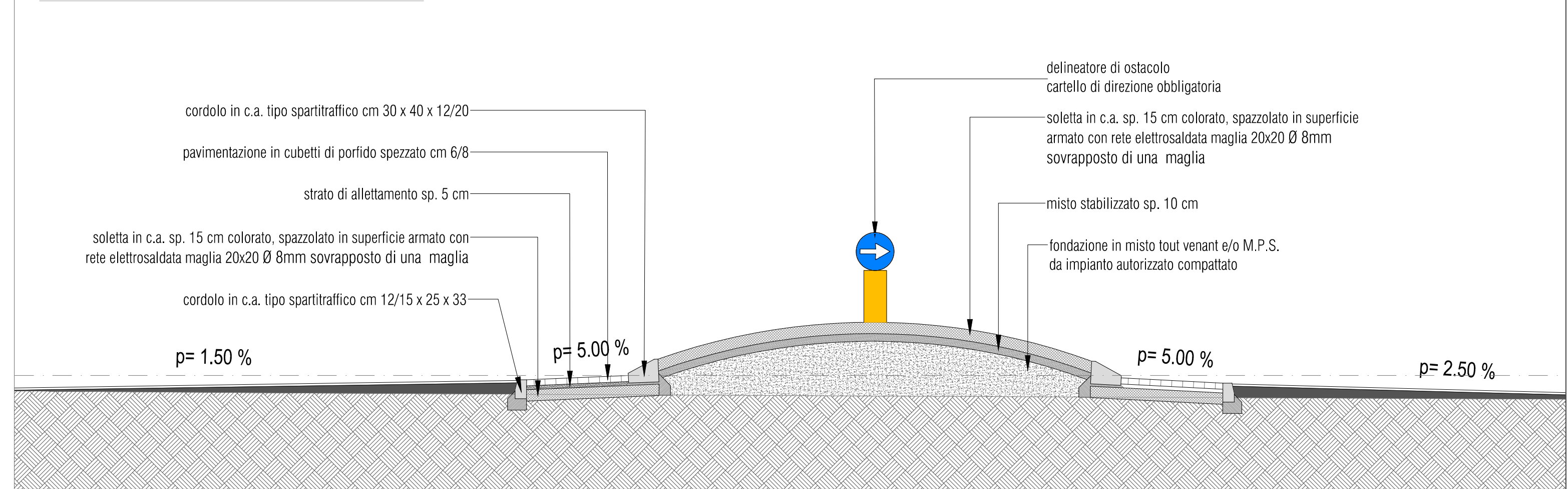
SEZIONE ISOLA CENTRALE - DETTAGLIO - Scala 1:50
