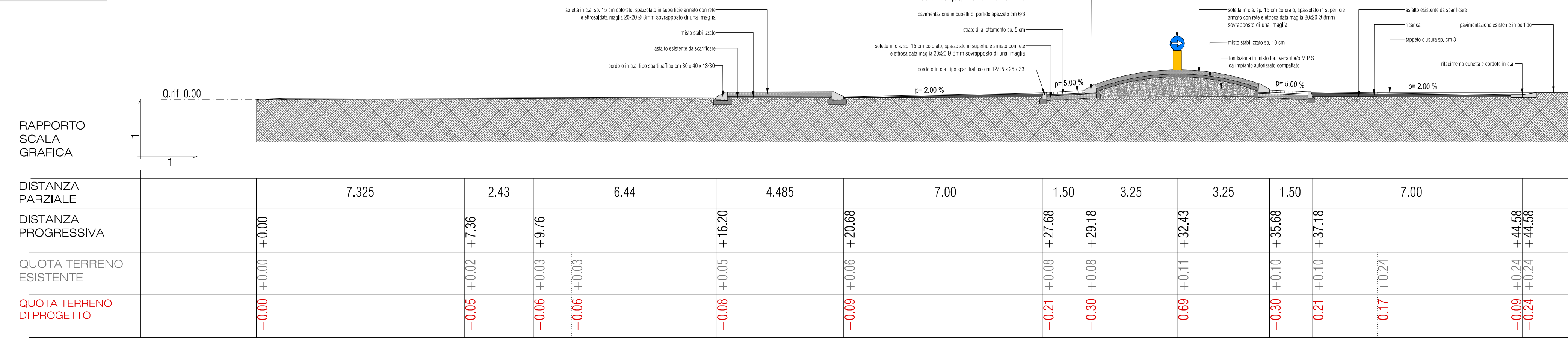
SEZIONE/PROFILO B-B - Scala 1:100
